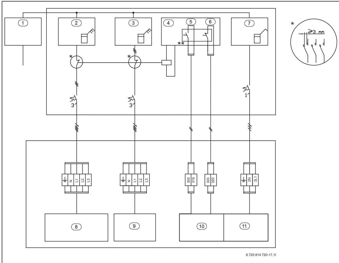
Kuva 29 EVU, tyyppi 1
