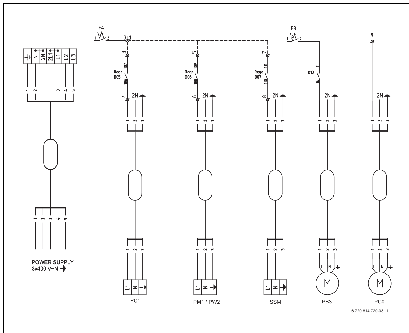
Kuva 17 Ulkoisten liitântöjen kytkentäkaavio, lämpöpumppu 54–80 kW
