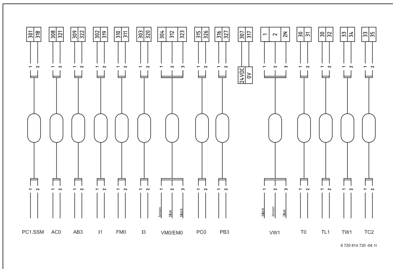
Kuva 18 Ulkoisten liitännöjen kytkentäkaavio, lämpöpumppu 54–80 kW
