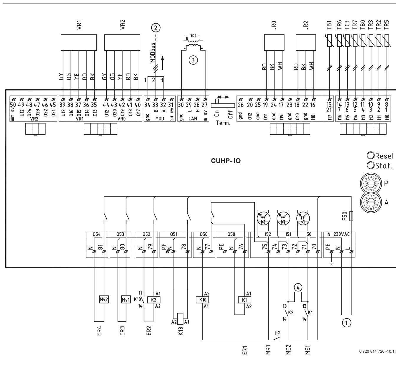
Kuva 26 Piirikaavio, lämpöpumppu 54–80 kW, koskettimella (K1/K2)
