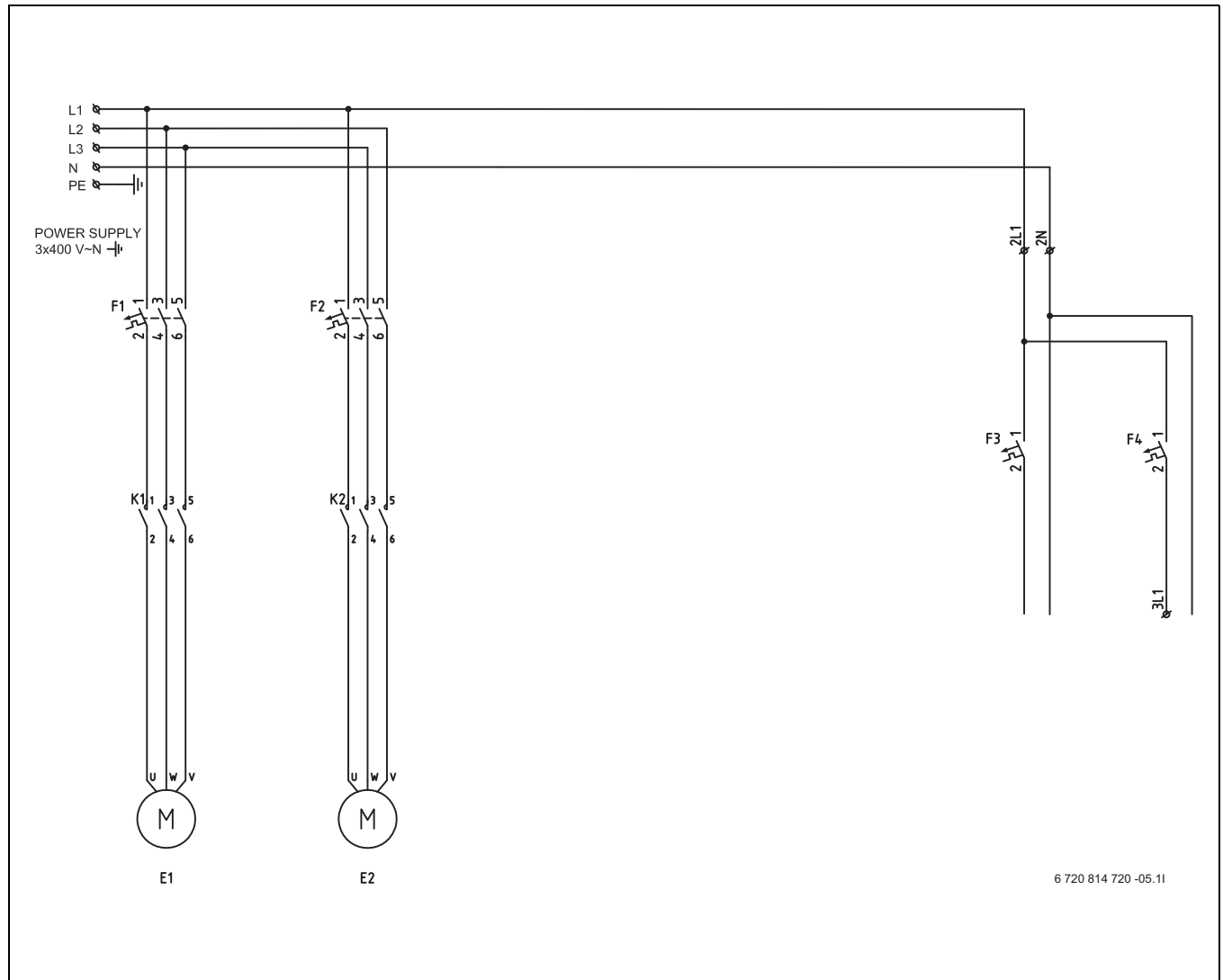
Kuva 20 Pääsyötön piirikaavio, lämpöpumppu 54–80 kW, koskettimella (K1/K2)
