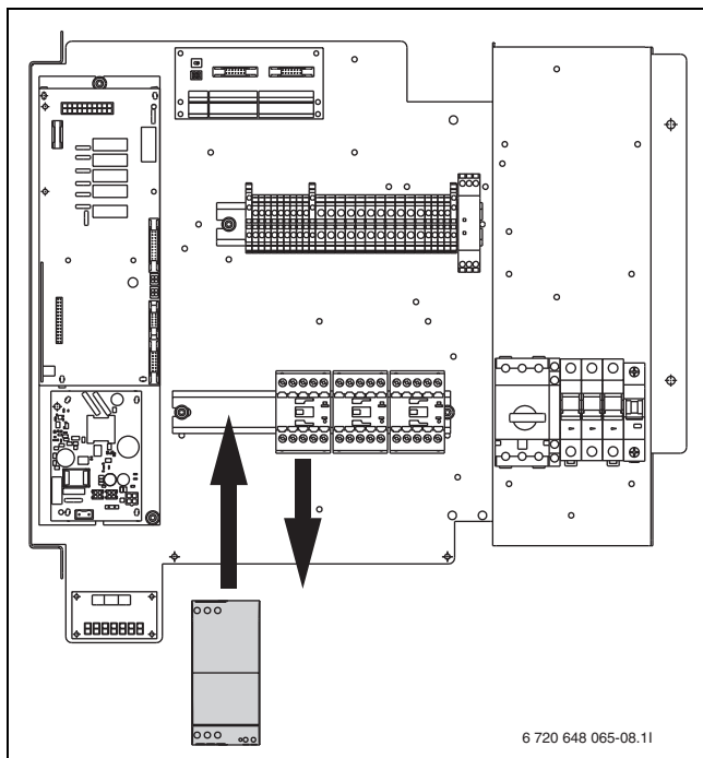
Kuva 33 Korvaa kontaktori
