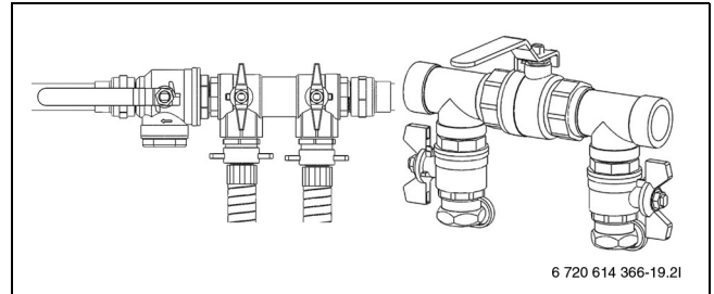
Kuva 22 Täyttösarjat täyttöasennossa
