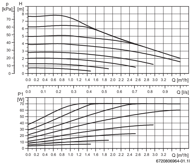
Kiertovesipumppu 6-9 LW
