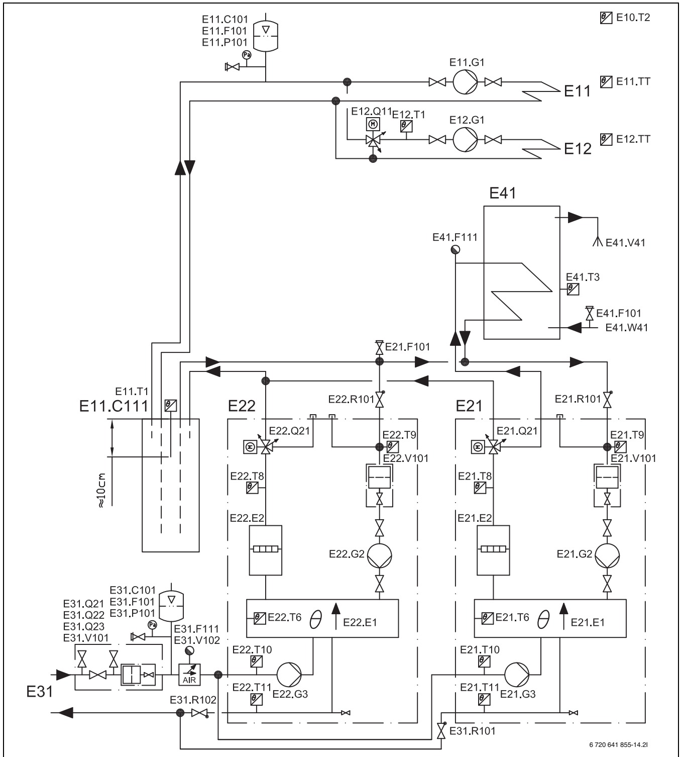
Kuva 61 Kaksi lämpöpumpua (kaskadiyhteyksellä), joissa shunttaamaton ja shuntattu lämmityspiiri, työväli ja ulkoinen käyttöveden lämmitys
