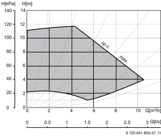
Lämmönkeruupumppu 11-17 LW
