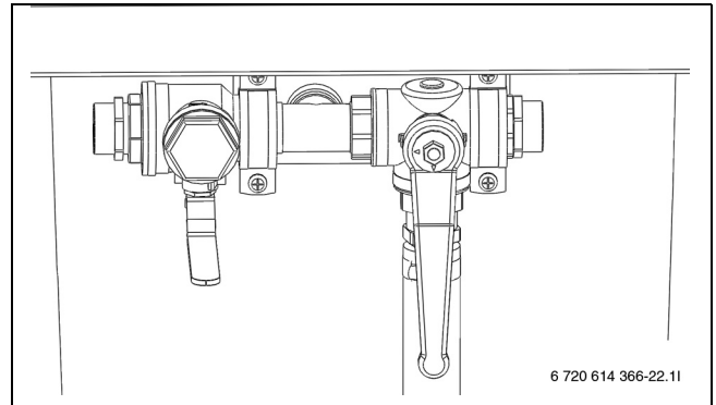
Kuva 23 Täyttöasema sekoitusasennossa
