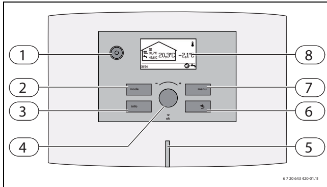
Kuva 46 Käyttöpaneeli
