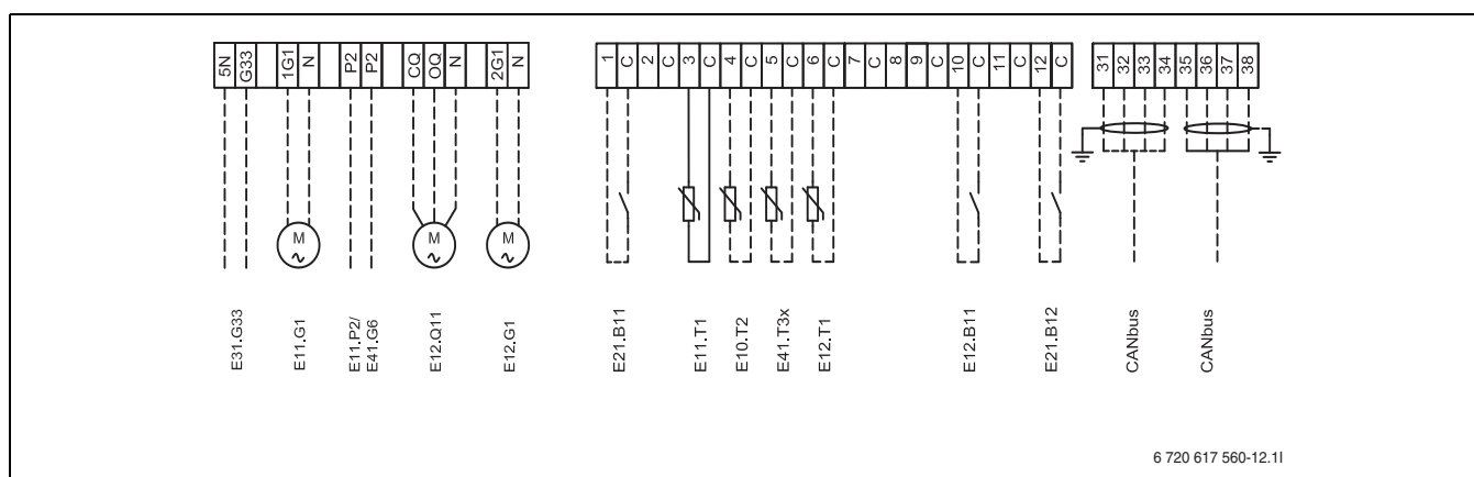
Kuva 44 Ulkoiset liitännät
