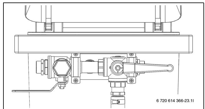
Kuva 24 Täyttöasema täyttötasennossa
