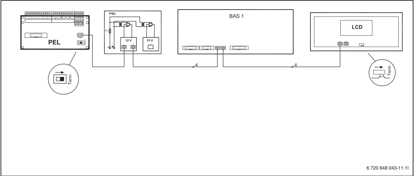
Kuva 39 CANBus, yleiskatsaus
