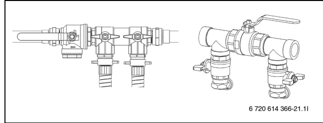
Kuva 26 Täyttösarjat normaaliasennossa
