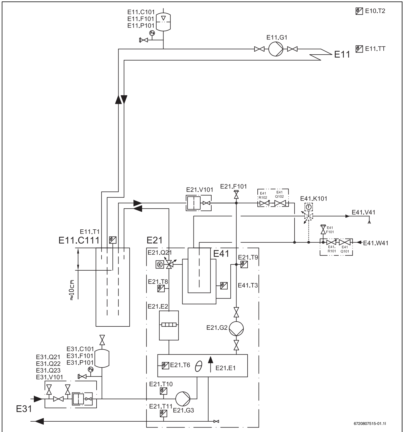
Kuva 10 Shunttaamaton lämmityspiiri ja työsäiliö
