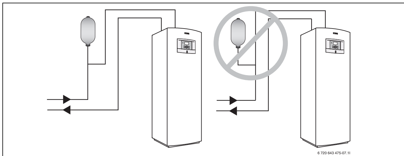
Kuva 15 Paisuntasäiliön asentaminen
