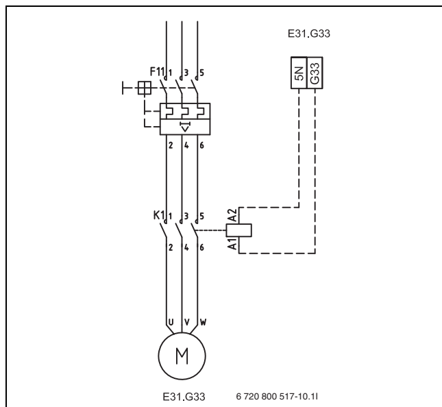
Kuva 45 Pohjavesipumpun liitäntä
