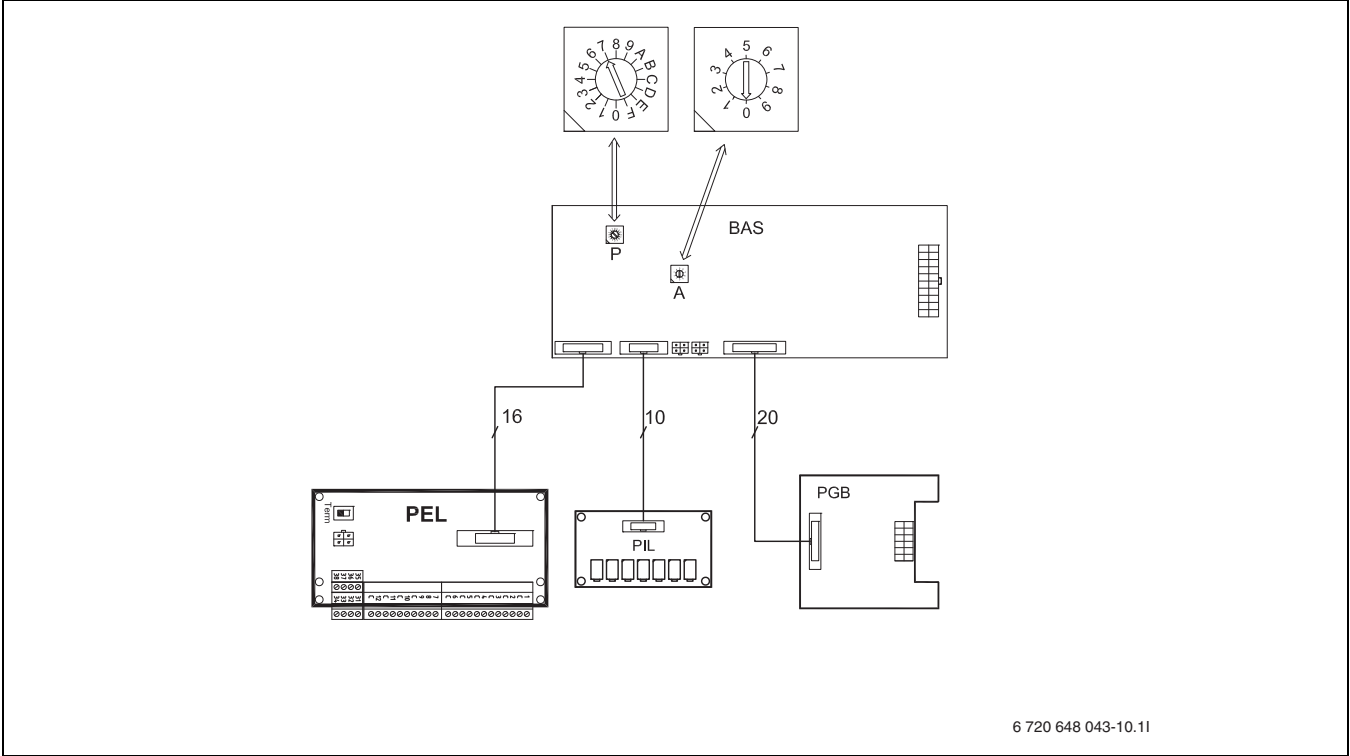
Kuva 40 Piirikortin johdotus
