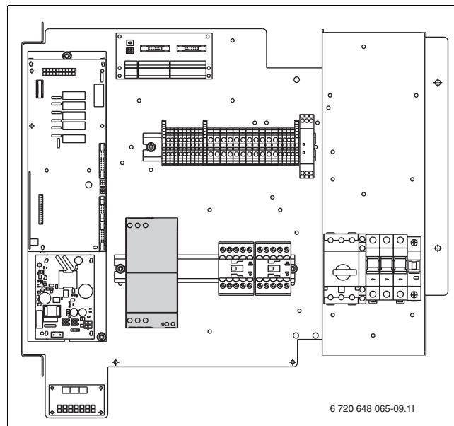
Kuva 34 Pehmökäynnistys asennettuna
