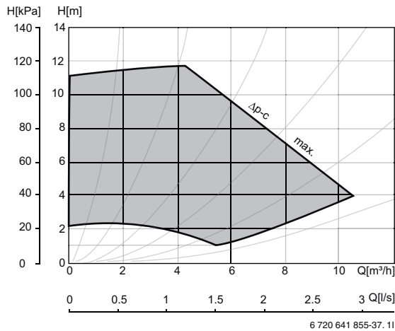
Lämmönkeruupumppu 11 LWM
