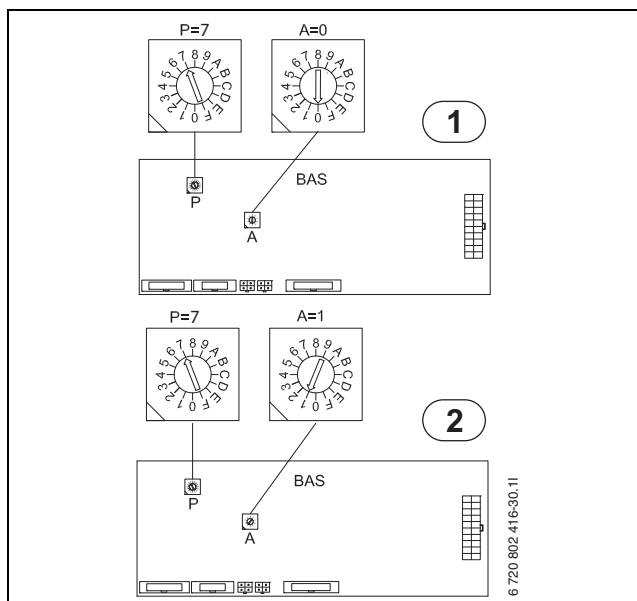
Kuva 63 Lämpöpumppujen 1 ja 2 säädöt kaskadiyhteyksessä.
