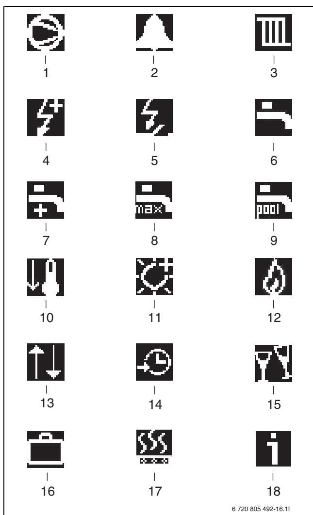
Bild 17 Driftsymboler
