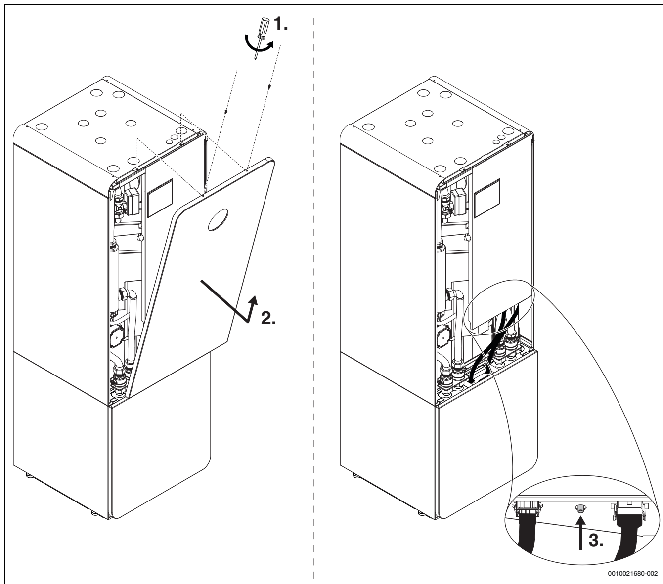
Bild 12 Återställning överhettningsskydd
