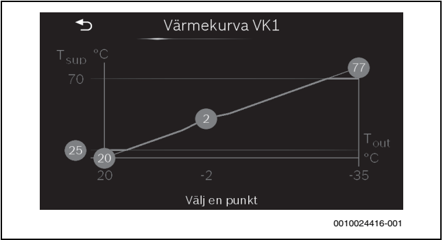
Bild 6 Utgångsvy värmekurva
