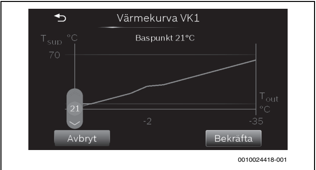
Bild 8 Justera baspunkt
