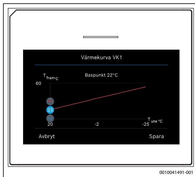
Bild 10 Justera baspunkt vid inställning med extra komfortpunkt
