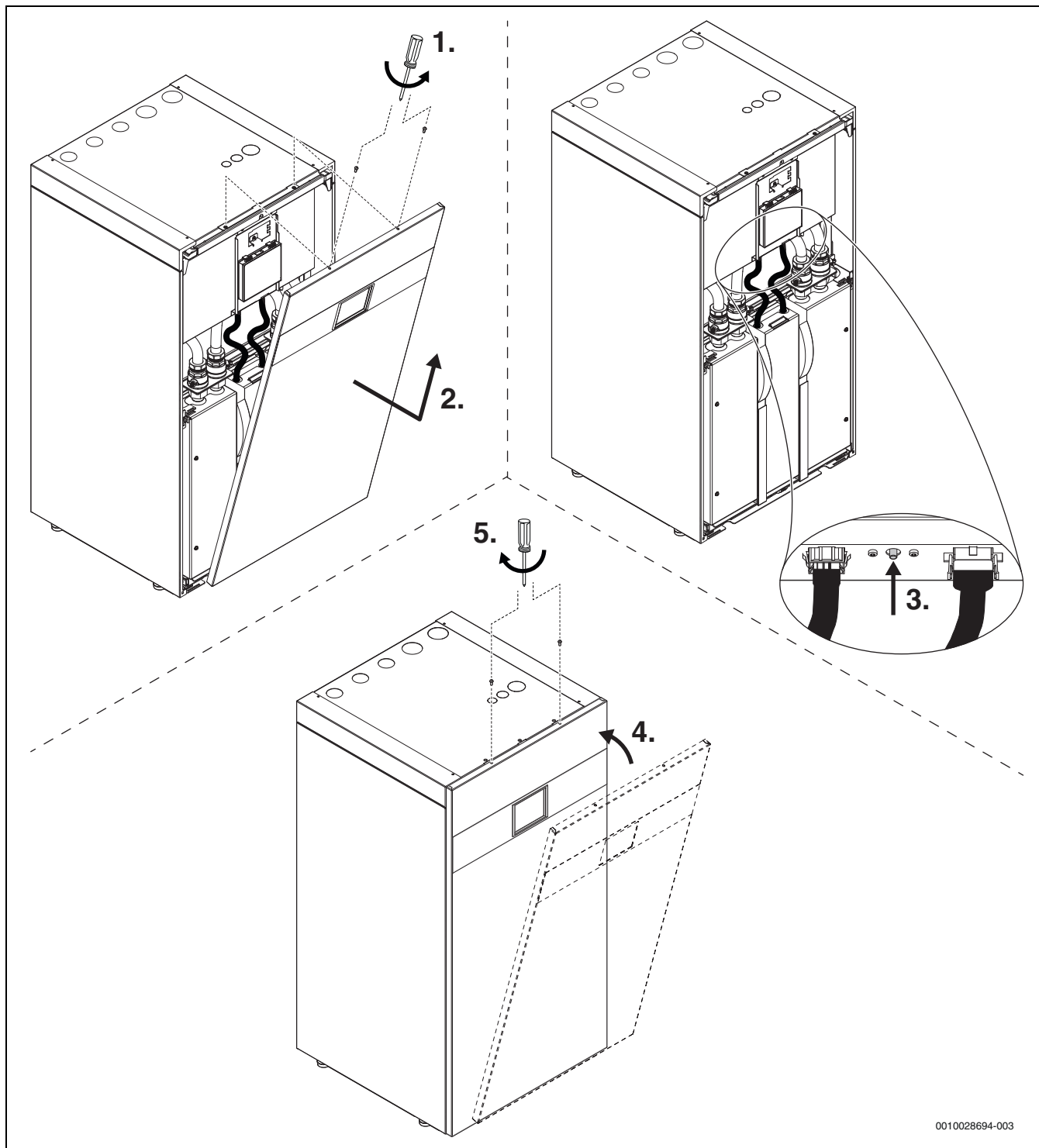
Bild 16 Återställning överhettningsskydd
