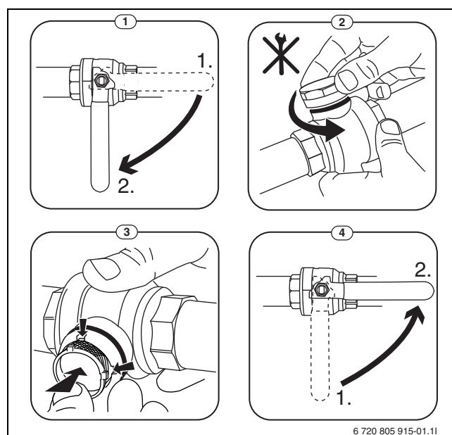
Bild 5 Filtrvariant utan låsring
