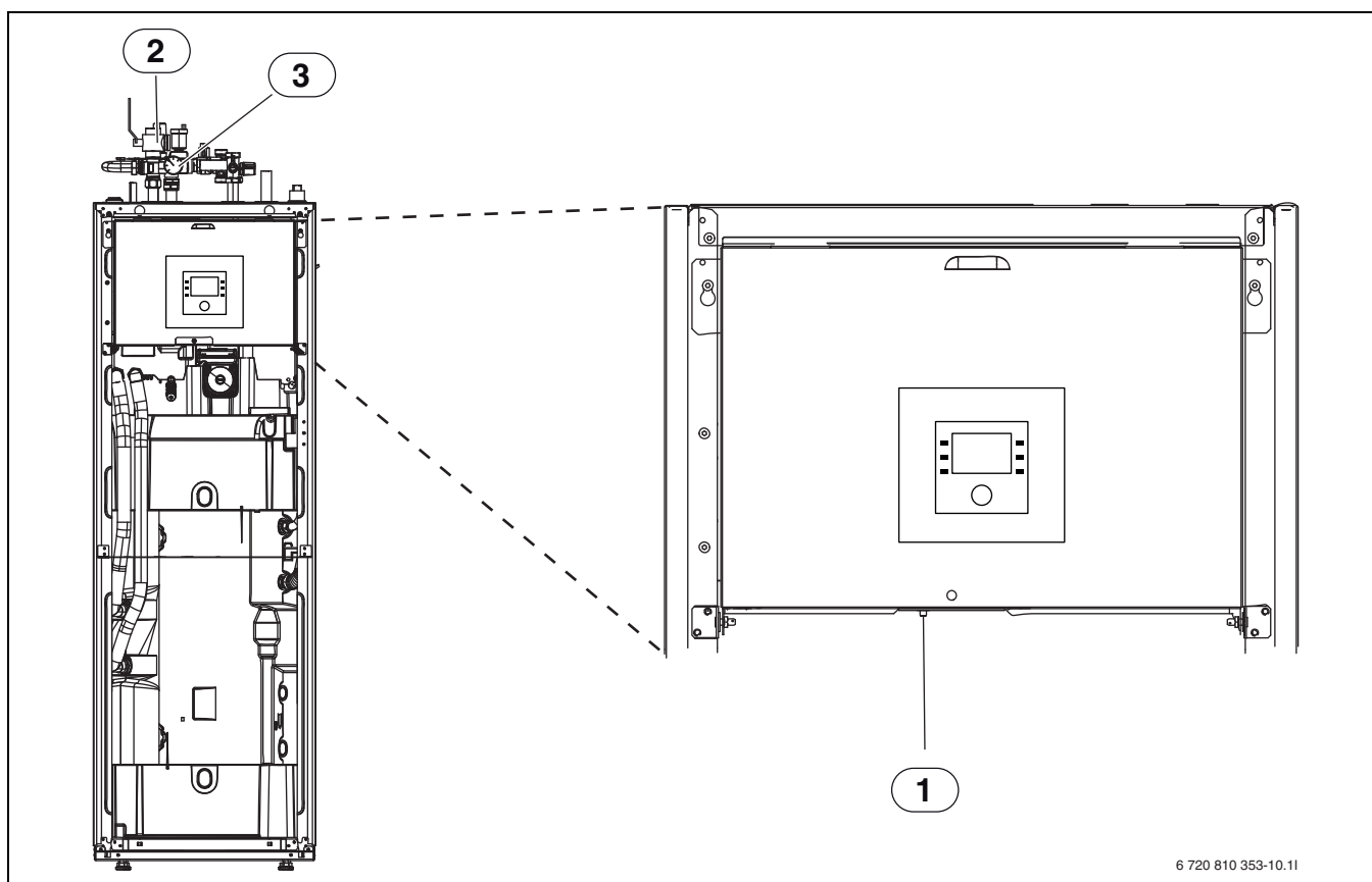
Bild 7 Inneenhet AWMS/AWMSS
