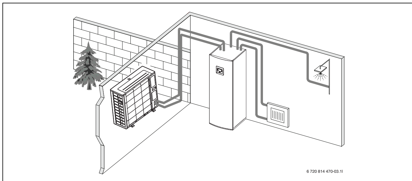
Bild 1 Värmepump (uteenhet), inneenhet AWMS/AWMSS med inbyggd varmvattenberedare och eltilskott
