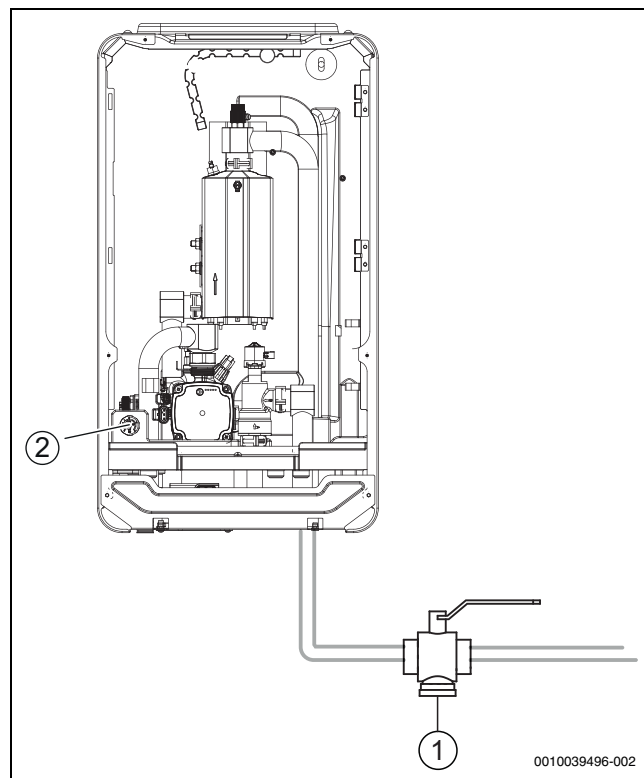
Bild 13 Inneenhet Compress 5800i 12 E
