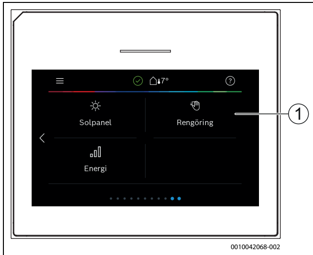
Bild 11 Reglercentral
