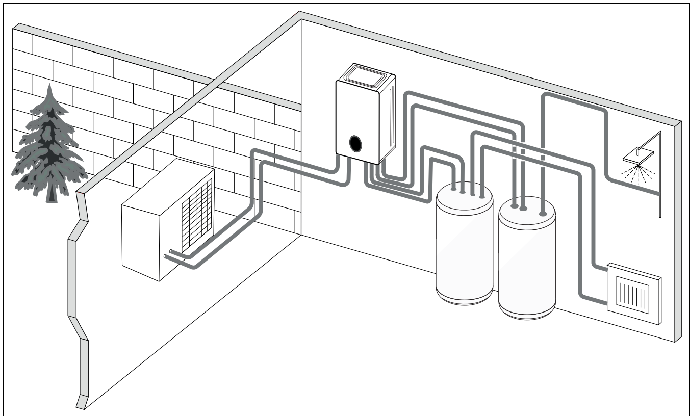
Bild 7 Värmepump AW OR, inneenhet Compress 5800i 12 E med el tillskott och extern varmvattenberedare
