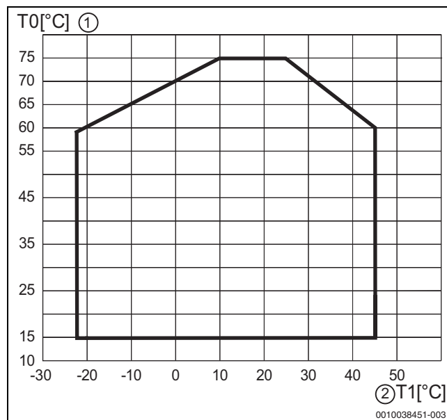
Bild 4 Värmepump i värmedrift utan tillskott
