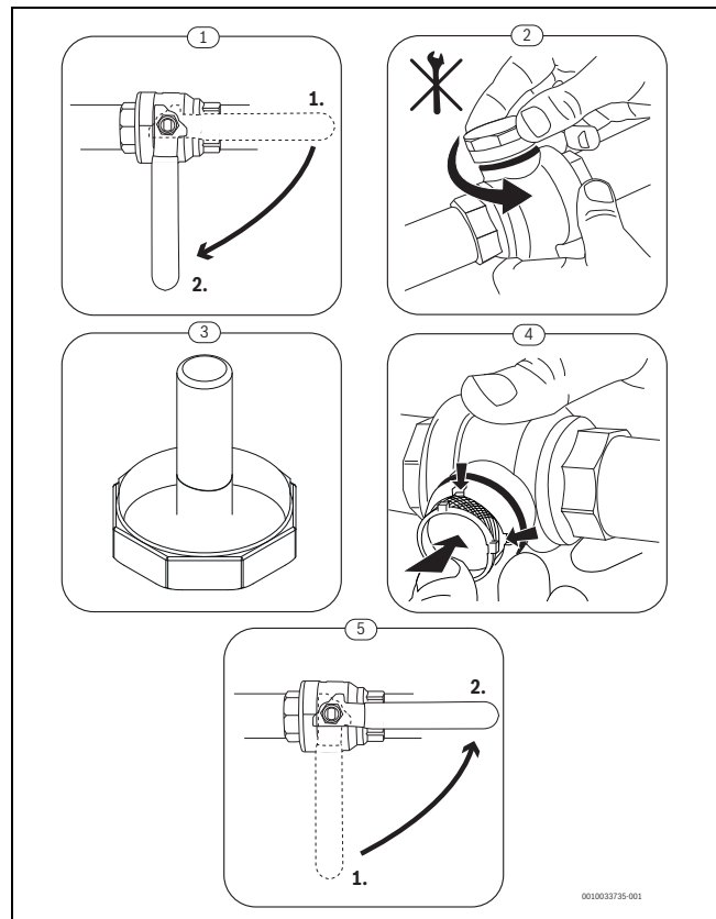
Bild 14 Rengöring av sil
