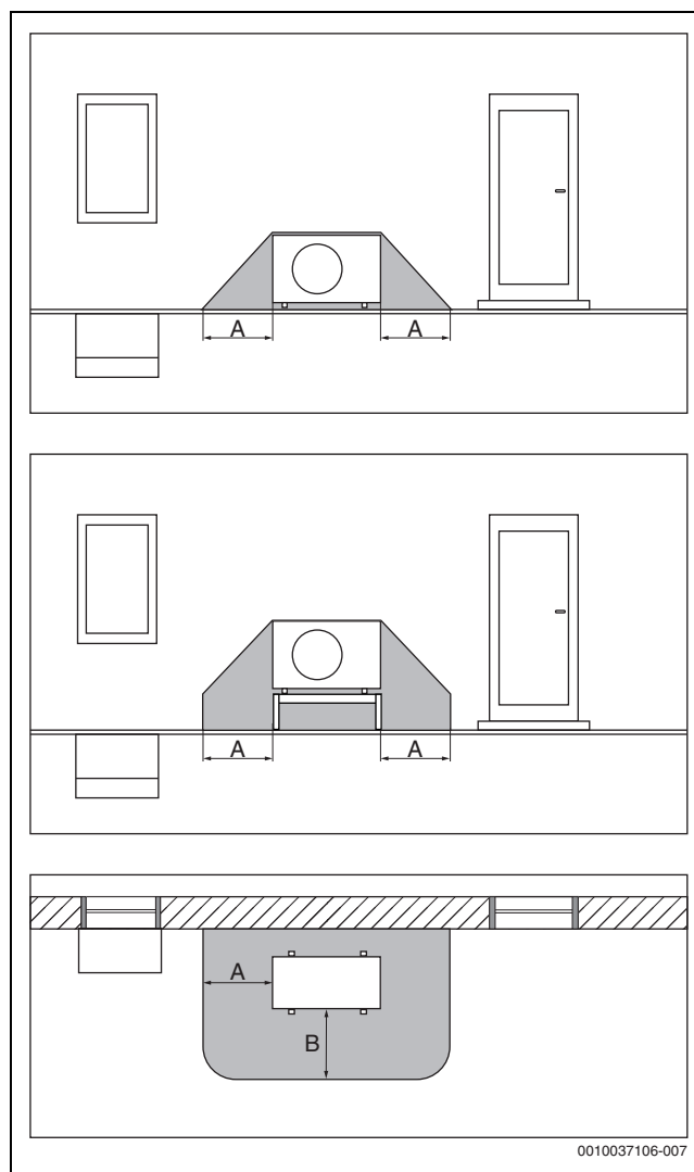
Bild 1 Skyddsområde markuppställd
