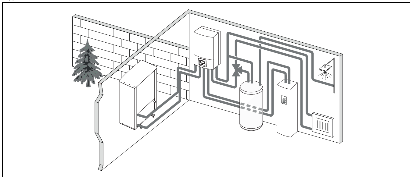
Bild 3 Värmepump Compress 7000 AW, inneenhet AWB utan eltilskott, extern varmvattenberedare och externt tillskott
