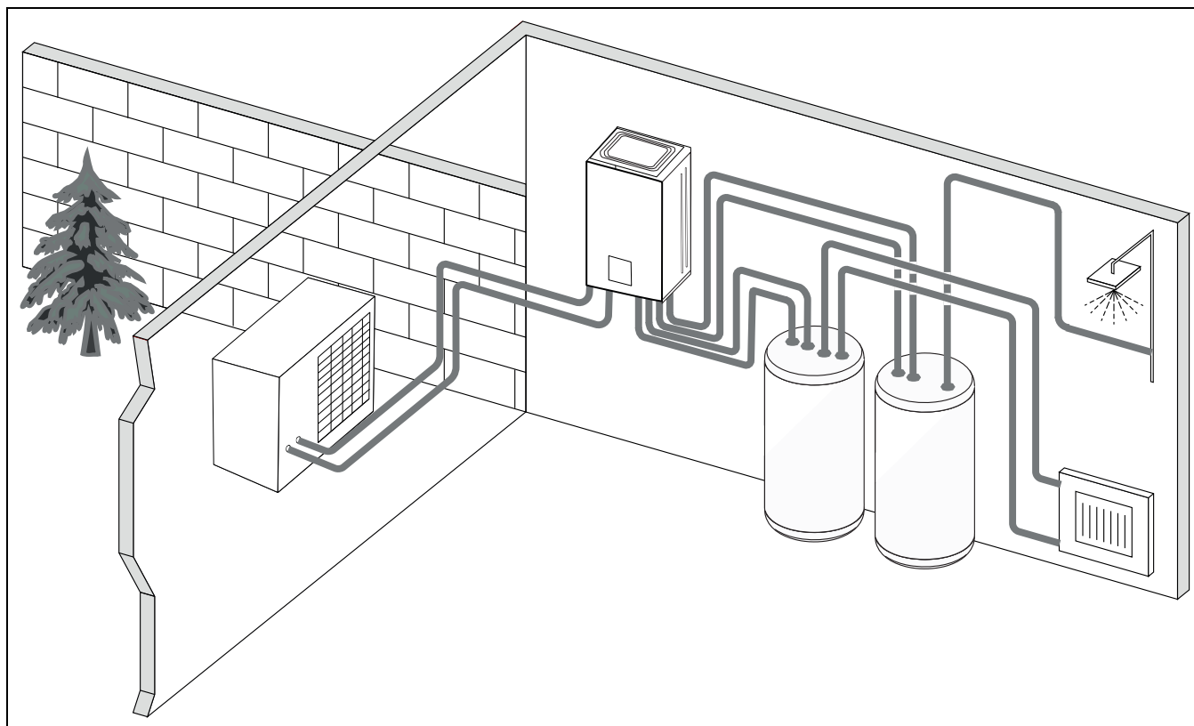
Bild 5 Värmepump AirX 500, inneenhet AirBox 500 E9 med eltillskott och extern varmvattenberedare
