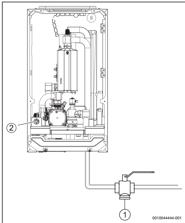
Bild 11 Inneenhet AirBox 500 E9
